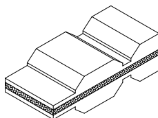
1-11/16" V-groove
